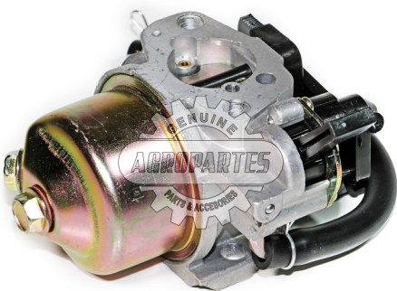
CARBURADOR GX160-200 GX160-27 SIN FILTRO
