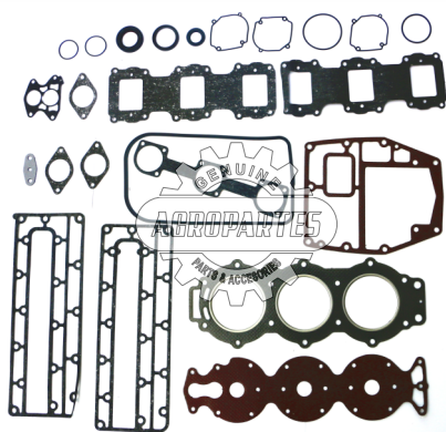
KIT EMPAQUES CABEZA FUERZA 75
